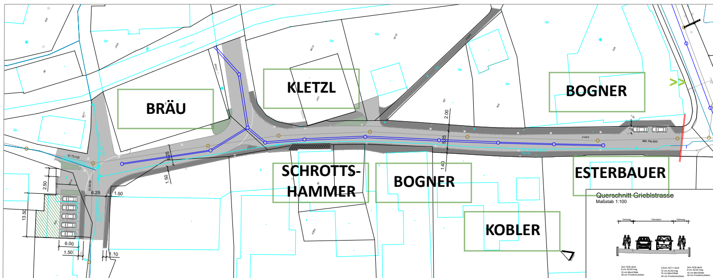
Plan von den Sanierungsarbeiten in der Griebelstraße / Schulstraße (Plan: IBZ)
