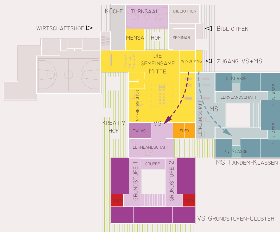
RAUMPROGRAMM EG
