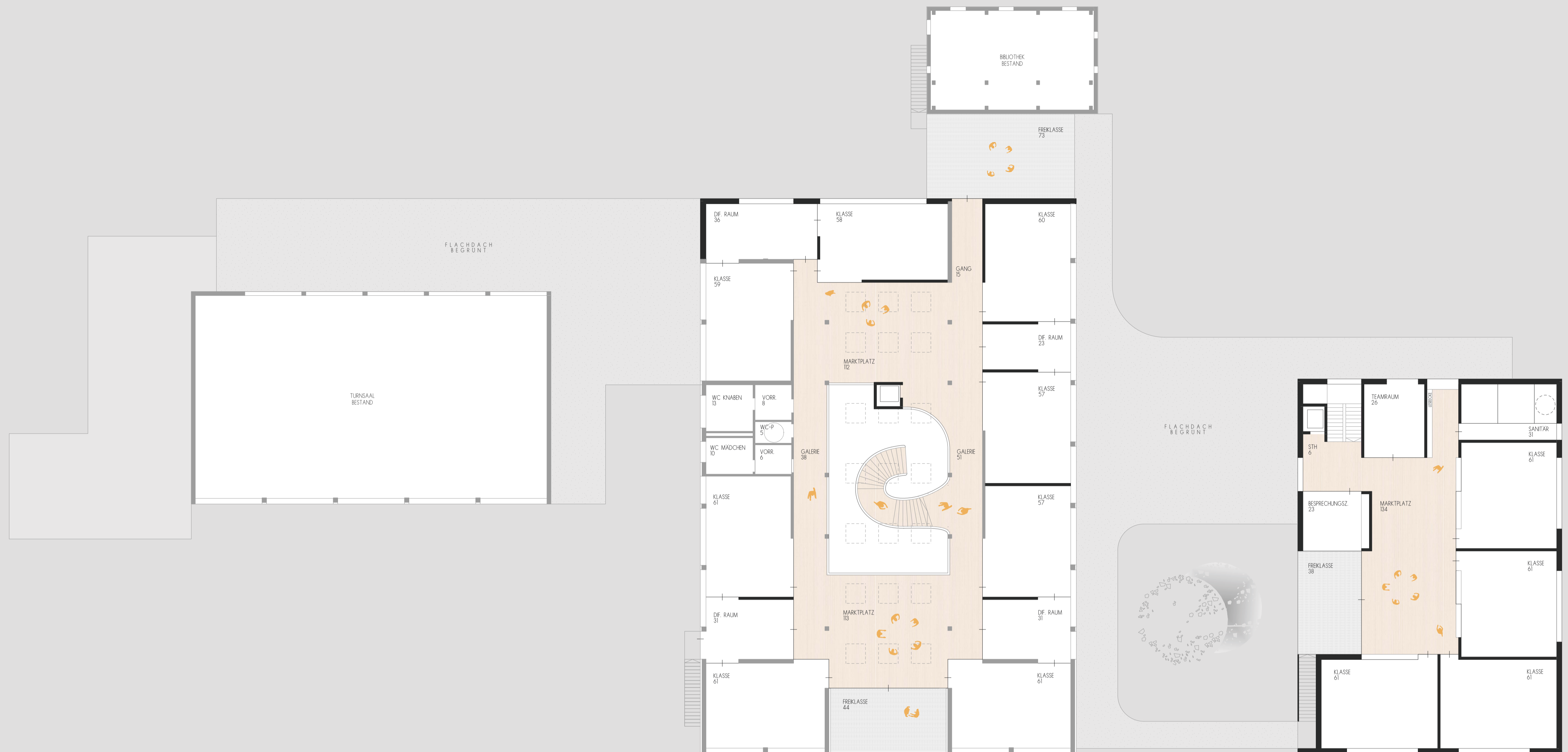
OBERGESCHOSS 1 | 200
