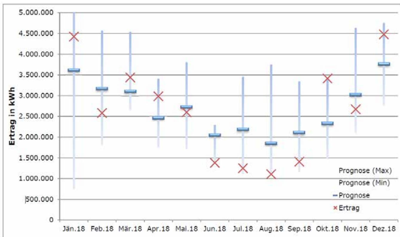
Winderträge Betriebsjahr 2018: --- Prognose laut Windgutachten X tatsächliche Erträge
